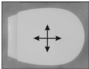
05 Verificare il corretto posizionamento del copriwater prima di serrare definitivamente il fissaggio. Check the correct position of the seat cover. Before tightening the fixing screw
