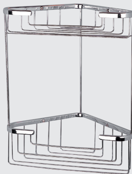
HÖRNKORG 655C Tvåplans, förkromad B250 x D150 x H310 mm
